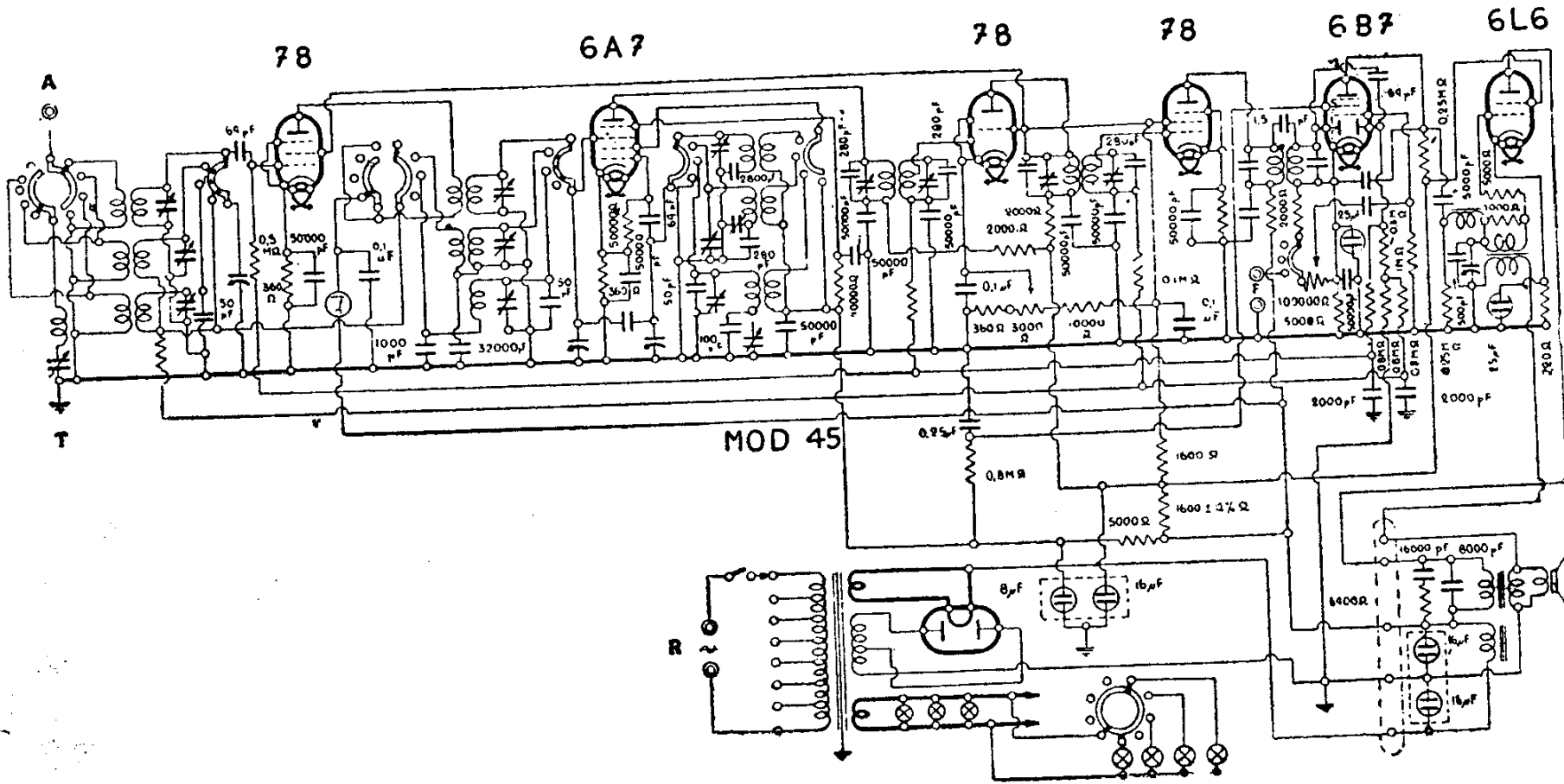
RADIO MARELLI . MOD. « MIZAR »
